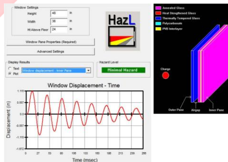
شکل ۱۶ شیهه سازی انفجار شیشه در نرم افزار
