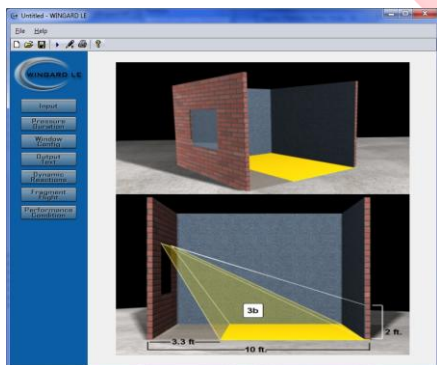
شکل ۱۶ شیهه سازی انفجار شیشه در نرم افزار
