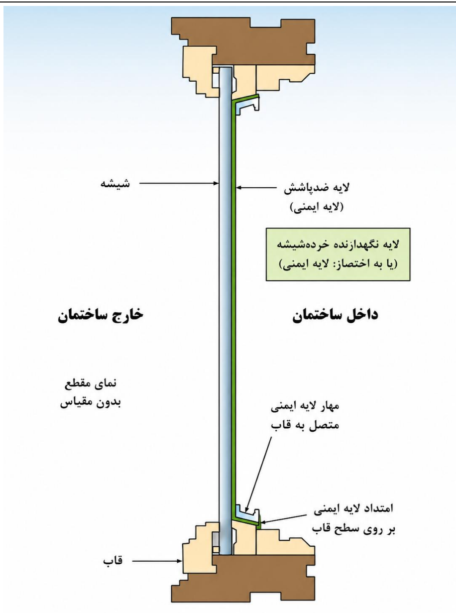
شکل ۱۸ لایه ایمنی شیشه (FRF) با مهار مکانیکی
