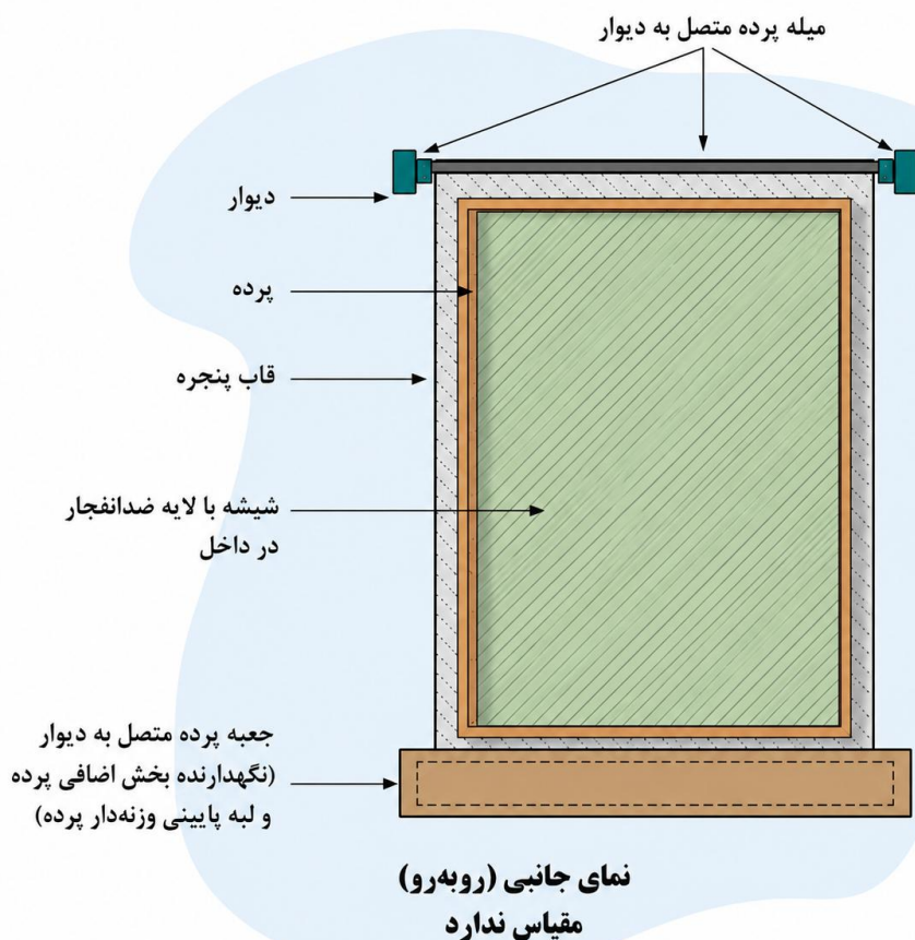
شکل ۲۱ سامانه پرده‌های مقاوم در برابر انفجار
