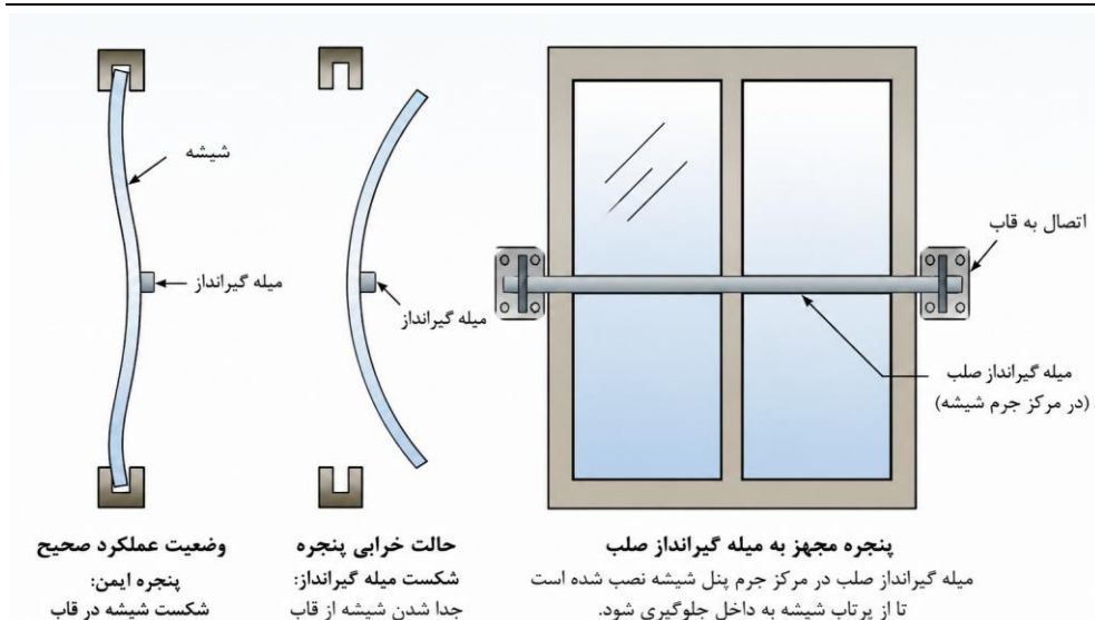
شکل ۱۹ شکل مفهومی سامانه میلۀ گیرانداز صلب
